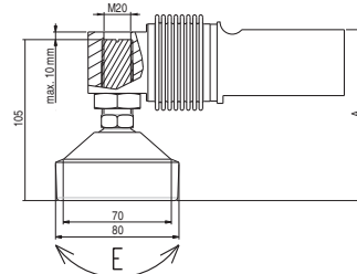
LFC 5 t
