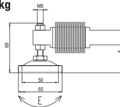
LFC 5 t
